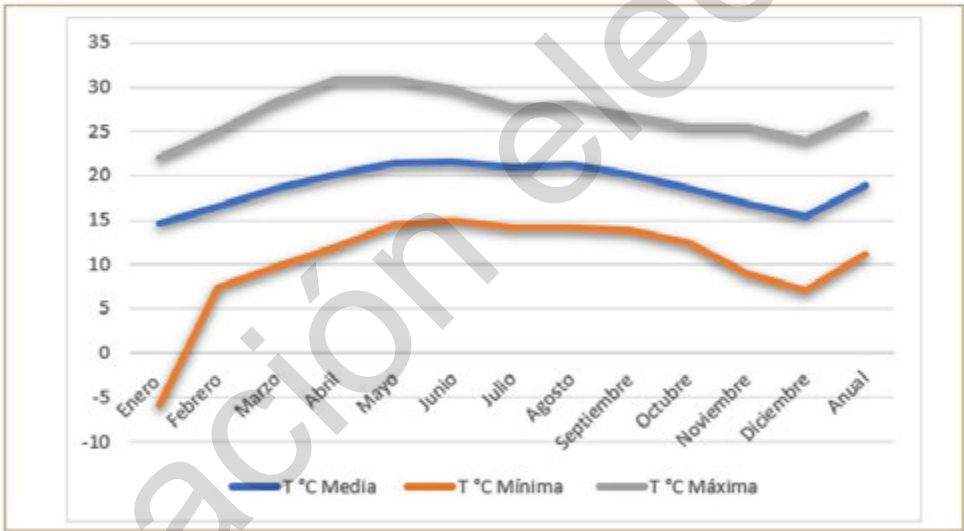
Figura 12. Gráfica Temperatura
